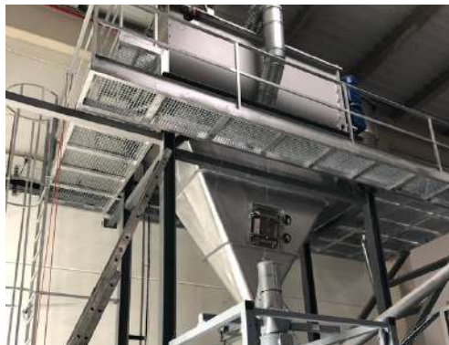
Mezcladora de cintas y tolva de descarga
