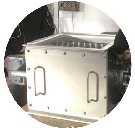
Rompe terrones
