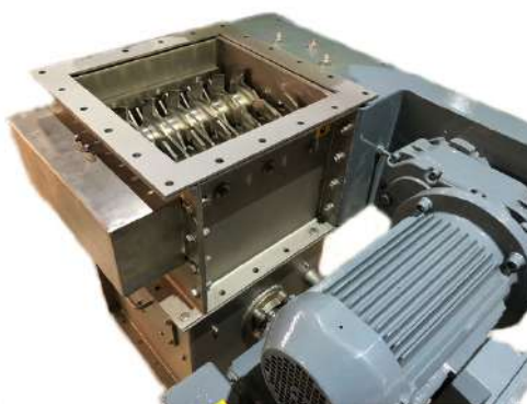
Conjunt desterronadors per additius
