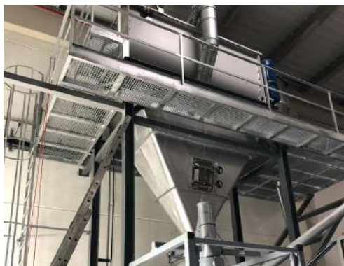
Barrejadora de cintes i tolva de descàrrega
